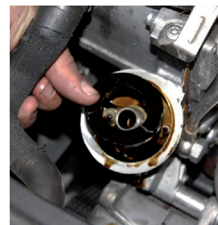
Рисунок 4: Старая прокладка может приклеиться к фланцу — ее следует обязательно удалить.
